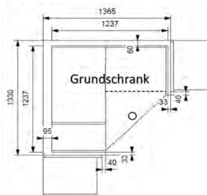
Begehbare Ecke, vollnutzbar, 2-türig
