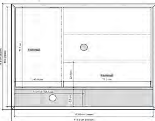
Paneel schwenkbar links oder rechts
